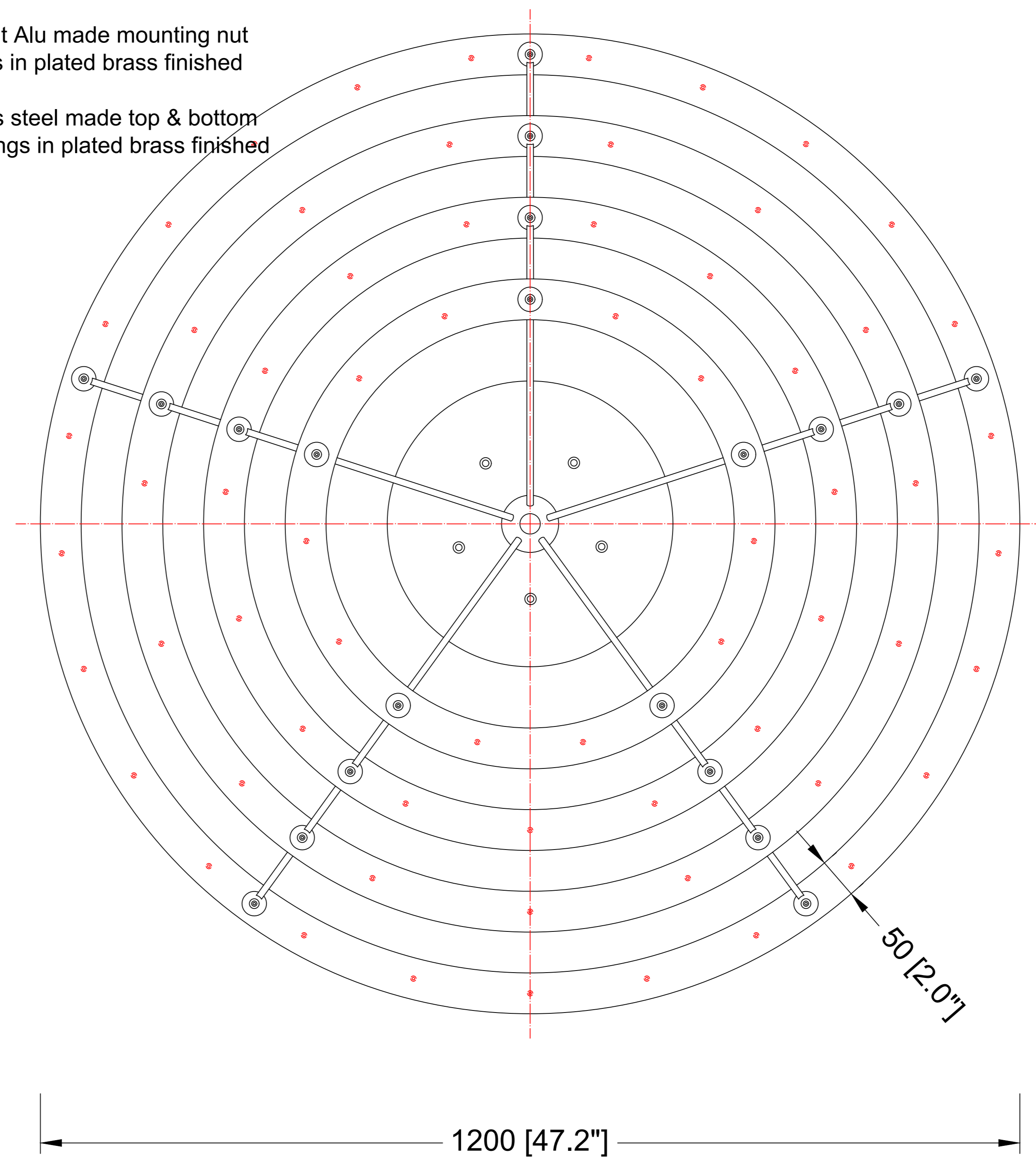
BOTTOM VIEW SCALE: 1:15
