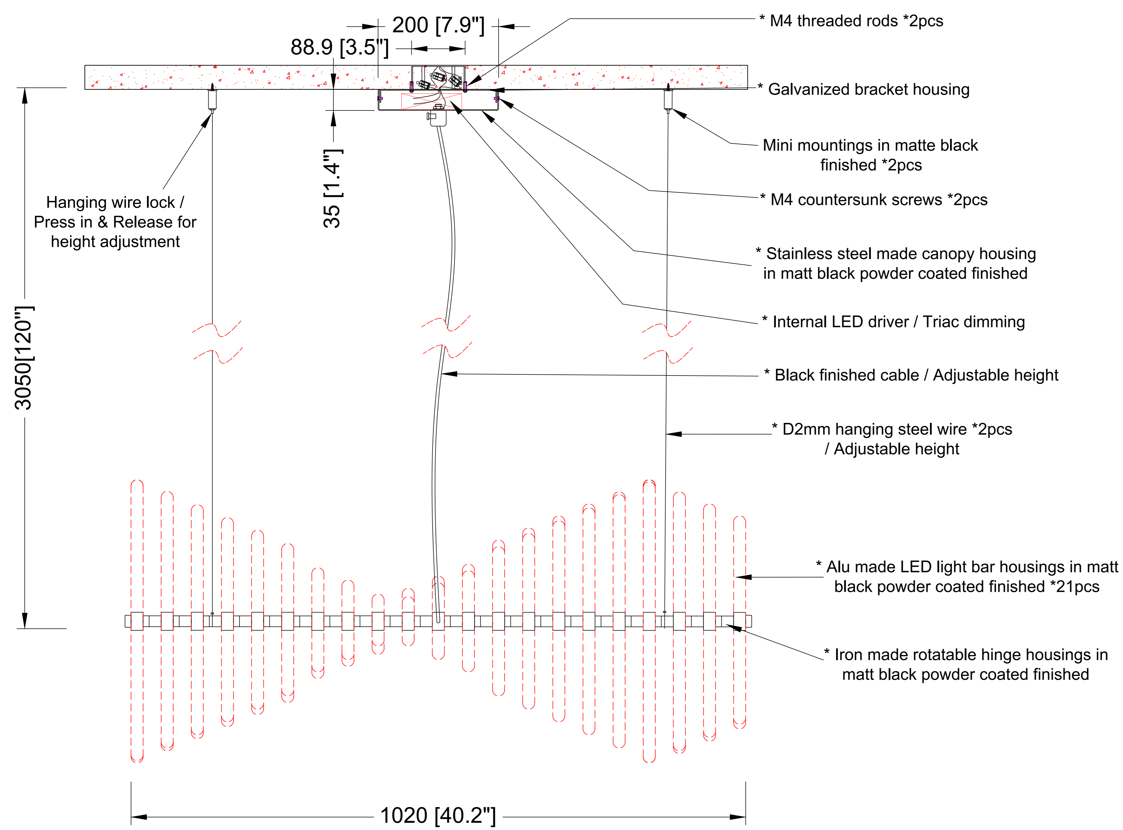
ELEVATION VIEW SCALE: 1:10
