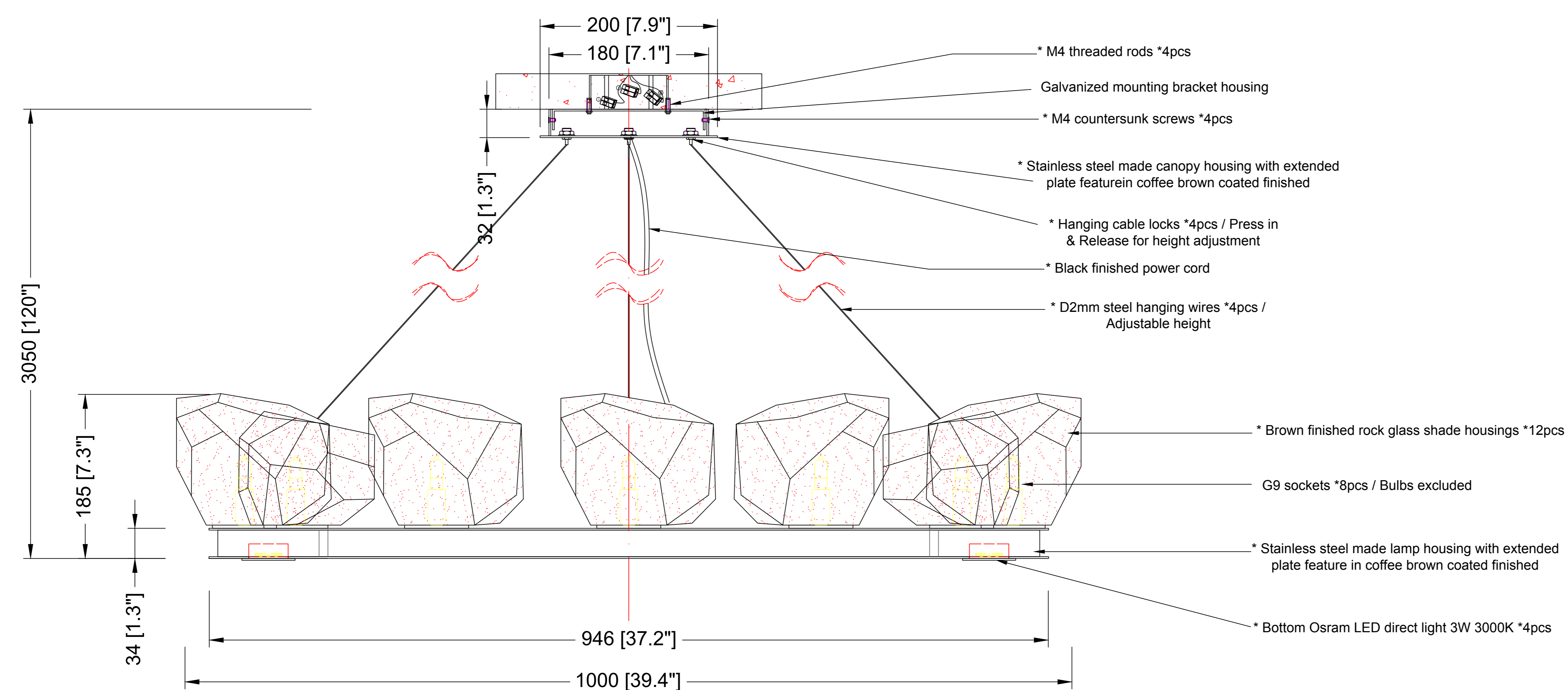
ELEVATION VIEW SCALE: 1:10
