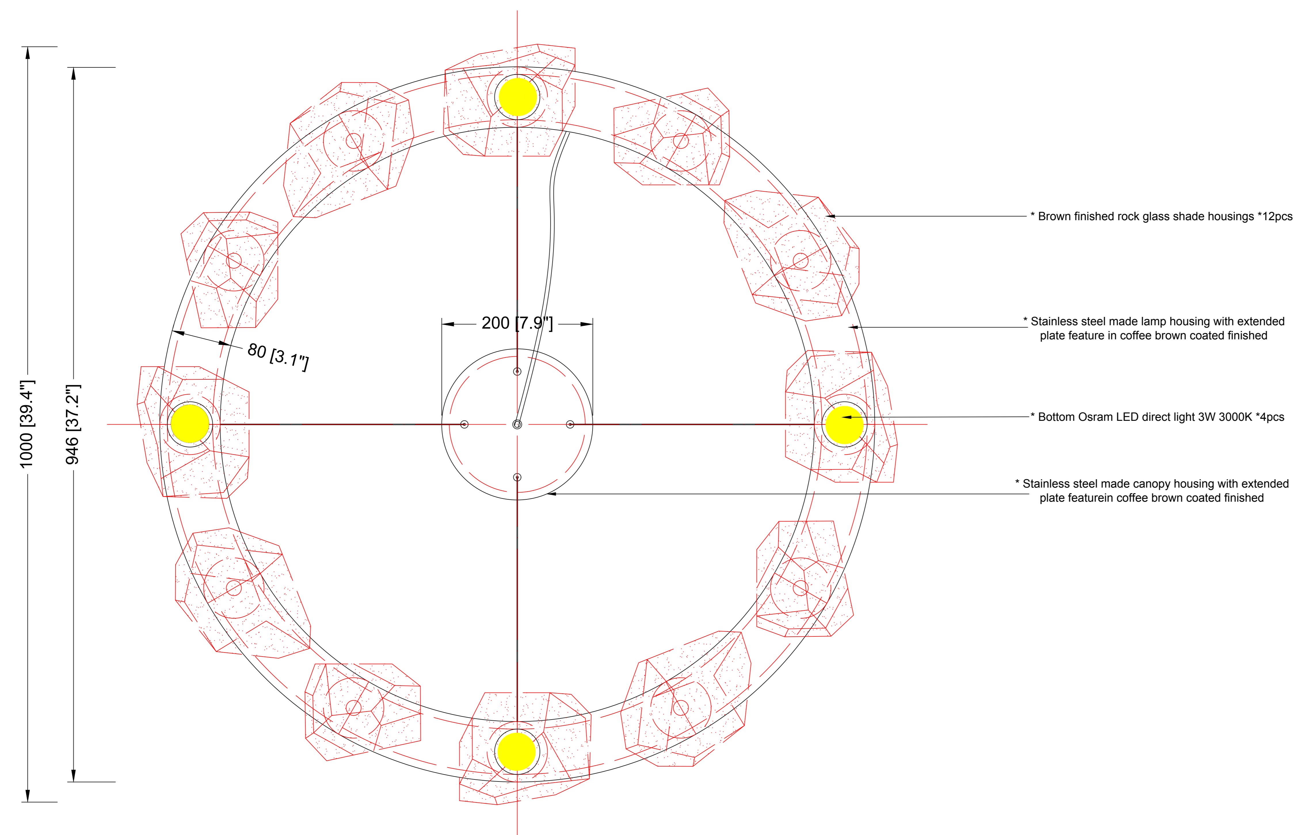
BOTTOM VIEW SCALE: 1:10
