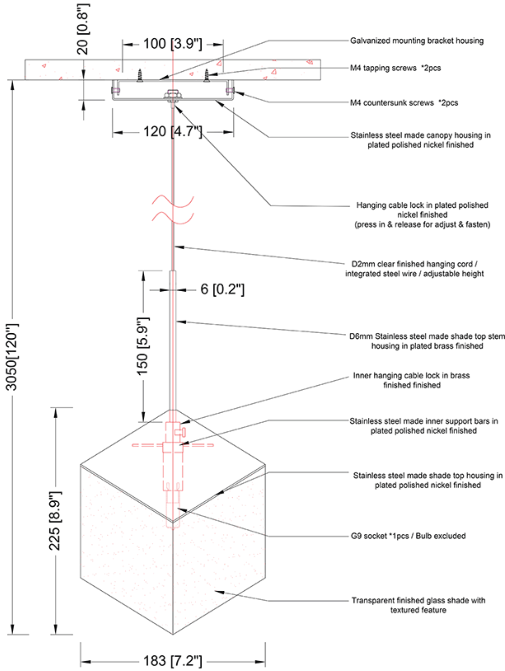
ELEVATION VIEW SCALE: 1:4
