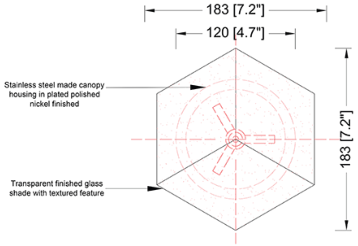
BOTTOM VIEW SCALE: 1:4
